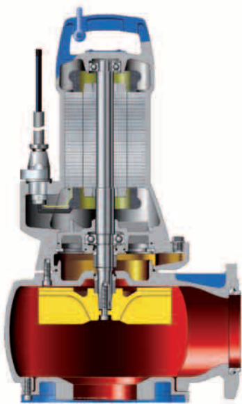
Rys. Przekrój zatapialnej pompy ściekowej KRT
